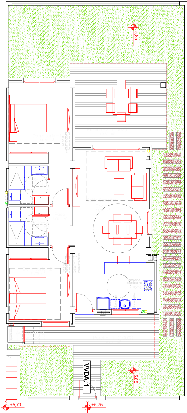
PLANTA BAJA.
