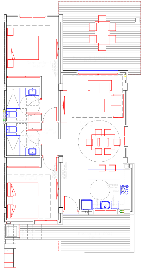
PLANTA BAJA.
